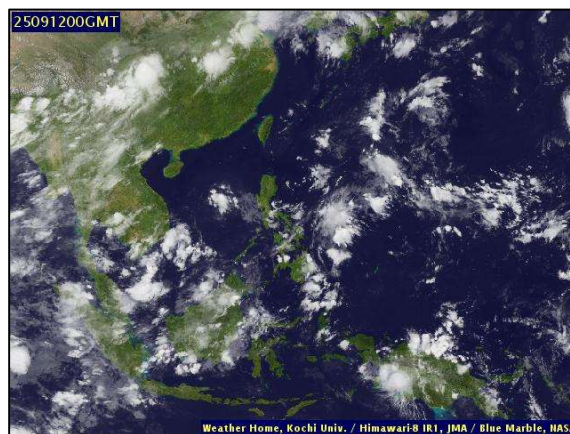
ภาพถ่ายดาวเทียม วันที่ ๑๒ ก.ย. ๒๕๖๘ เวลา ๐๗.๐๐ น.
